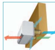
Luftfluß bei AusbläÙ nach unten im Wärmepumpenbetrieb
