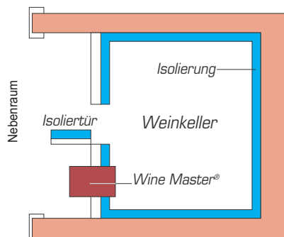
Installationsschema für C18, C18S und C50S
