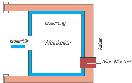
Installationsschema für C18SR und C50SR
